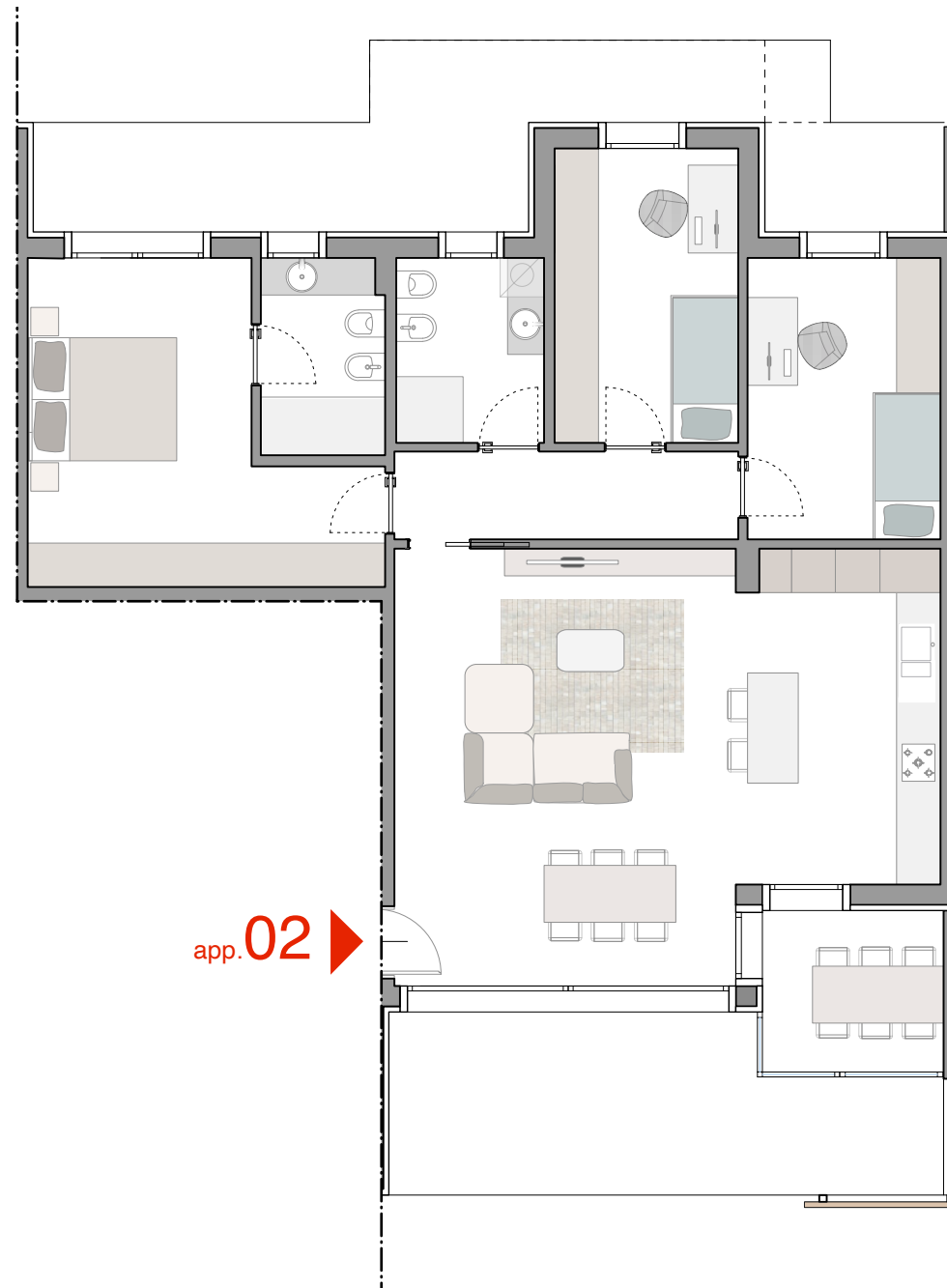
Pianta lay-out
