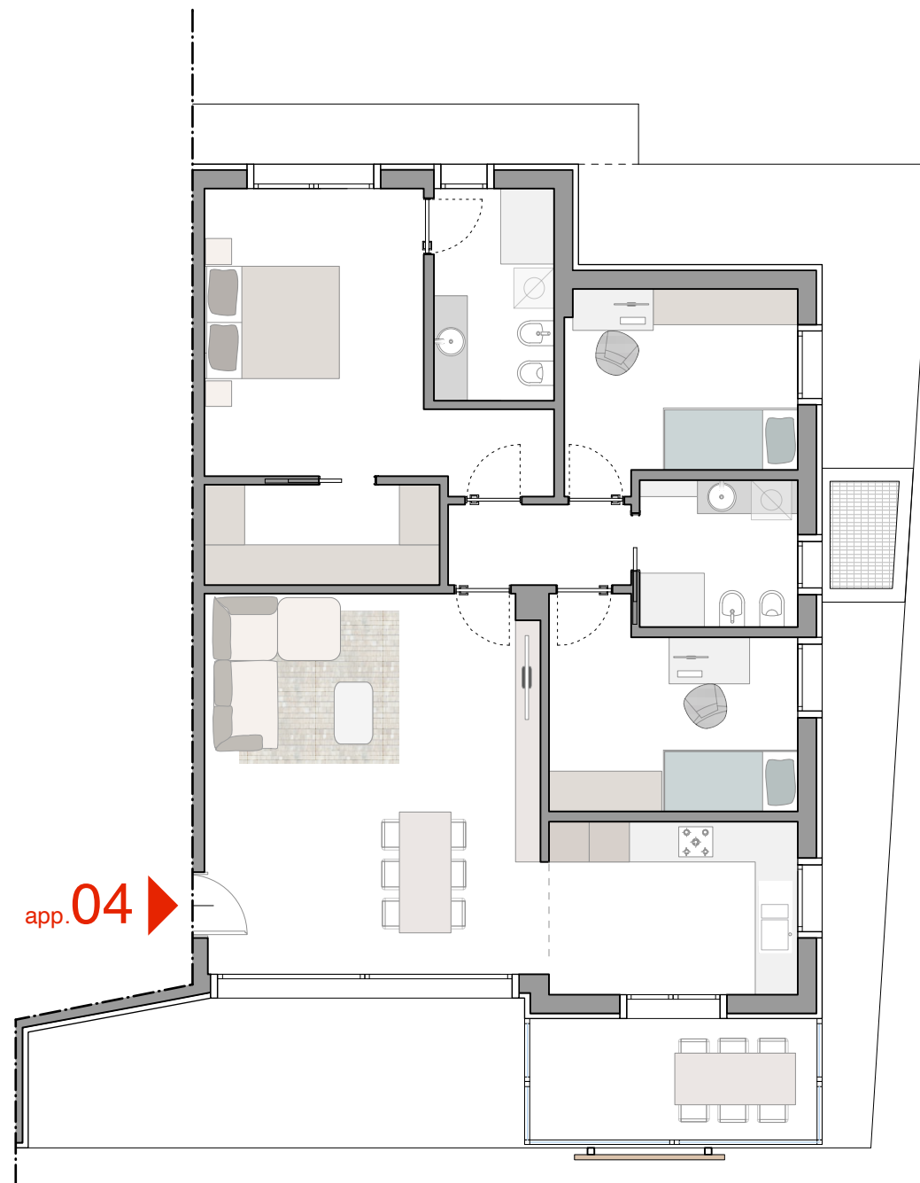
Pianta lay-out
