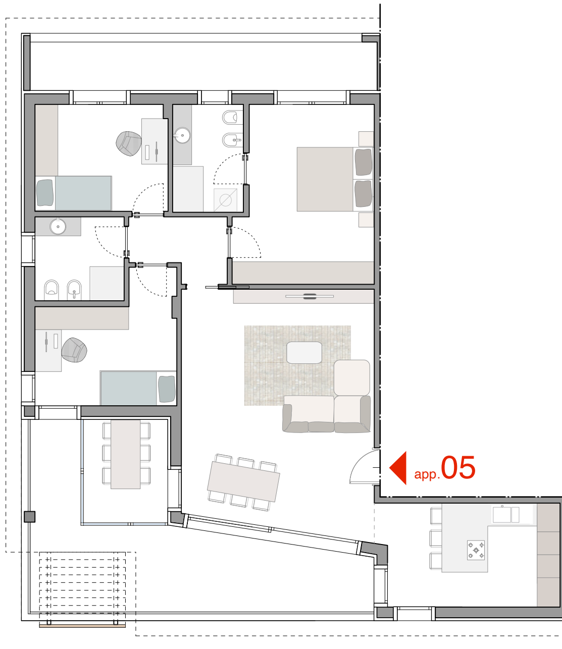
Pianta lay-out
