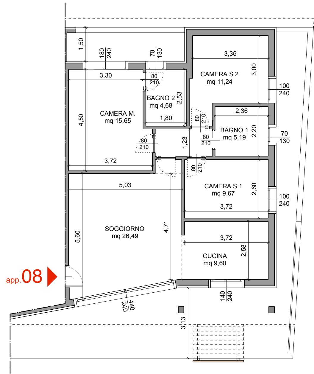
Pianta
